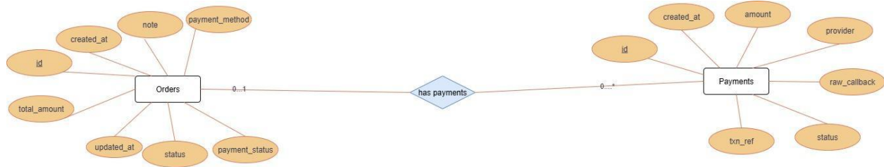
Hình 10. Mối quan hệ ERD giữa bảng Order và bảng Payment
