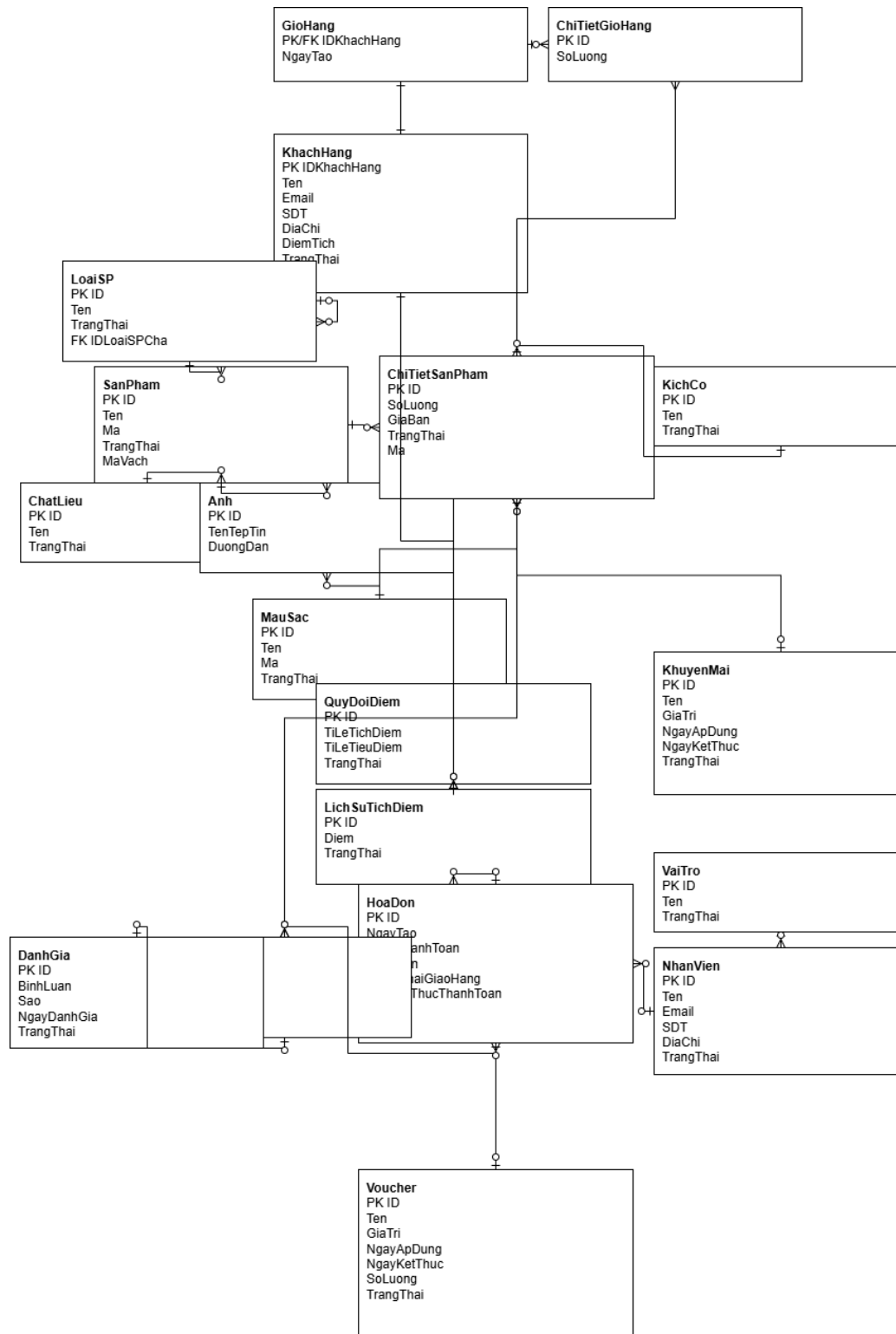
Hình 33. Sơ đồ ERD loại logical
