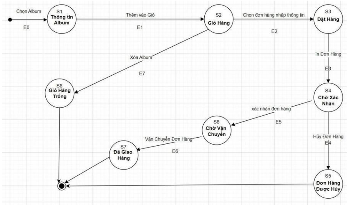
Hình 40. Kiểm thử trạng thái trong Kiểm thử hộp đen
