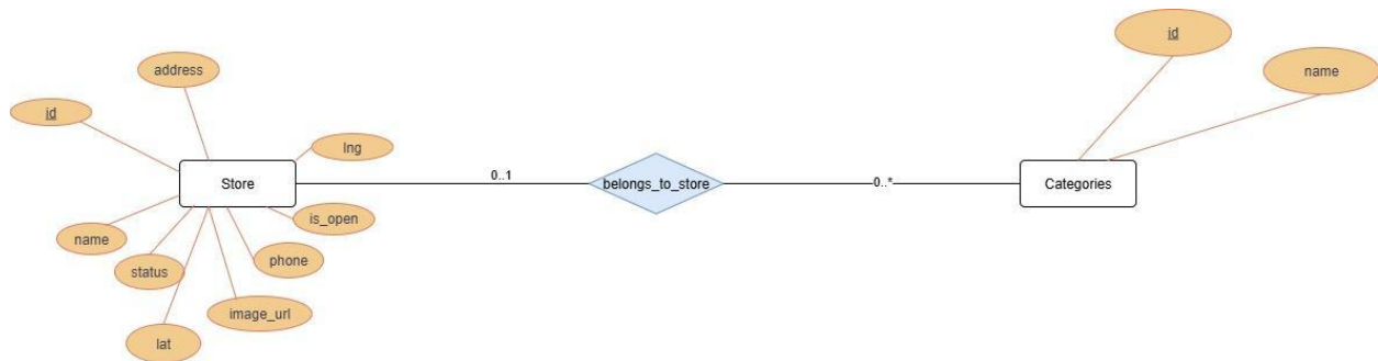
Hình 5. Mối quan hệ ERD giữa bảng Sore và bảng Category
