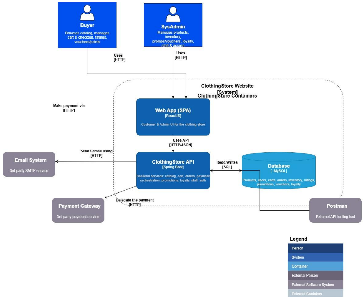
Hình 20. Hình vẽ C2 Container trong C4 model
