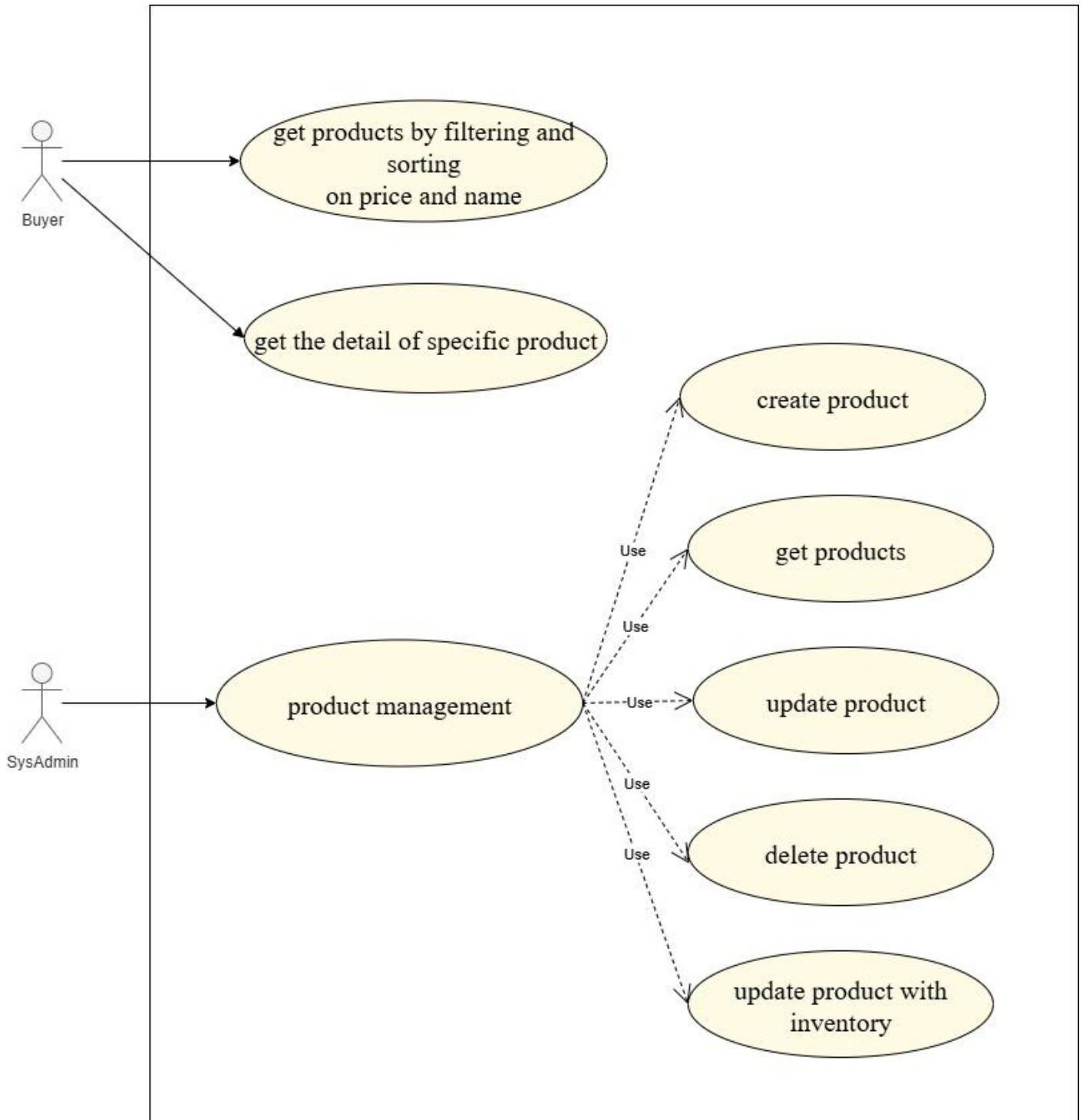
Hình 11. Draw the usecase of Product Catalog
