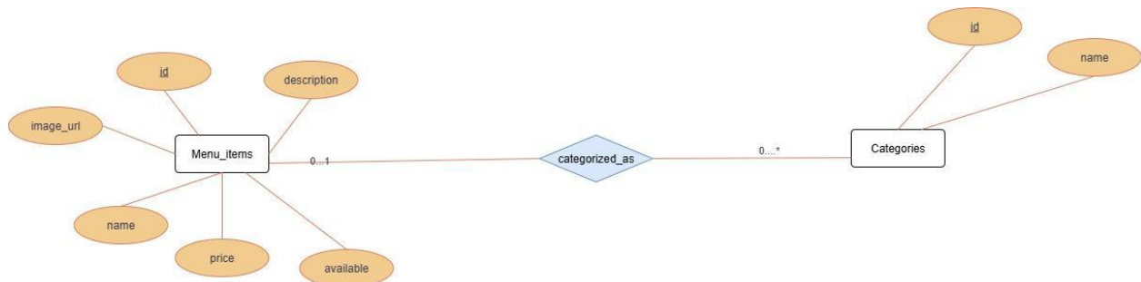
Hình 7. Mối quan hệ ERD giữa bảng MenuItem và bảng Category
