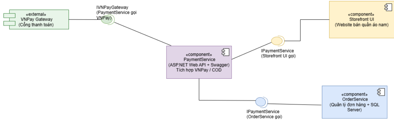
Hình 26. Component payment method (VNpay)
