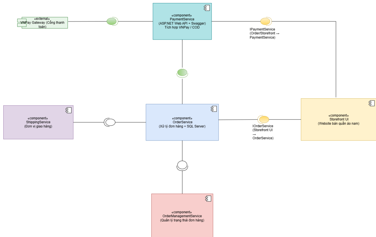
Hình 27. Component Clothes Orders
