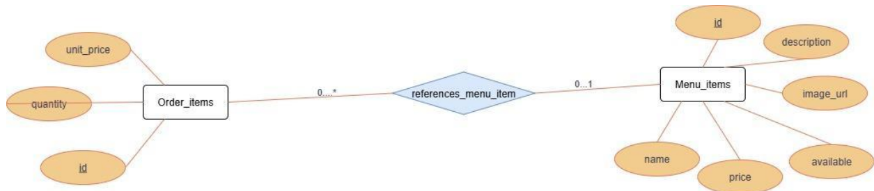
Hình 12. Mối quan hệ ERD giữa bảng OrderItem và bảng MenuItem
