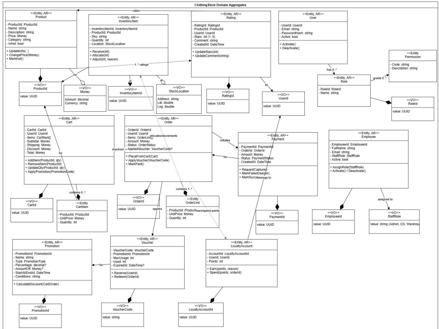
Hình 23. Hình vẽ C4 Code (clothing store aggregate) trong C4 model
