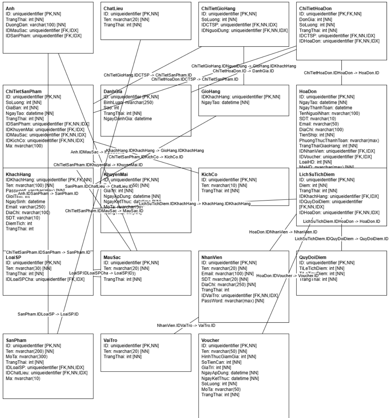
Hình 32. Sơ đồ ERD loại physical
