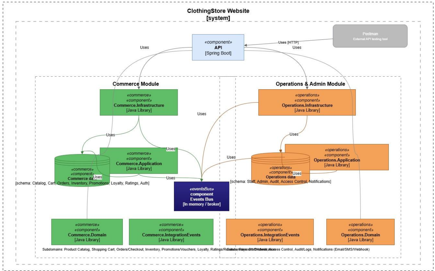
Hình 22. Hình vẽ C3 Component (module-level) trong C4 model
