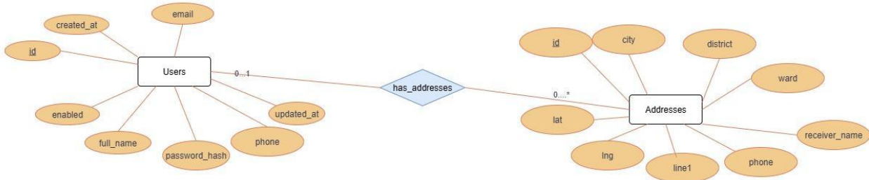
Hình 1. Mối quan hệ ERD giữa bảng User và bảng Address
