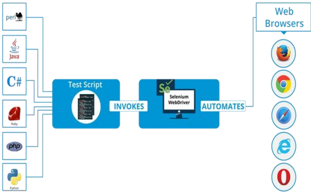
Hình 34. Hình ảnh minh họa thiết lập trong môi trường thử nghiệm
