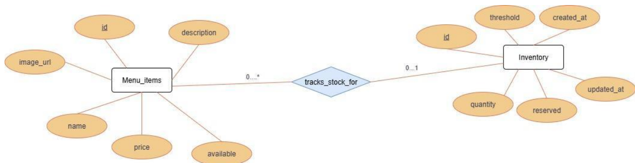
Hình 8. Mối quan hệ ERD giữa bảng MenuItem và bảng Inventory
