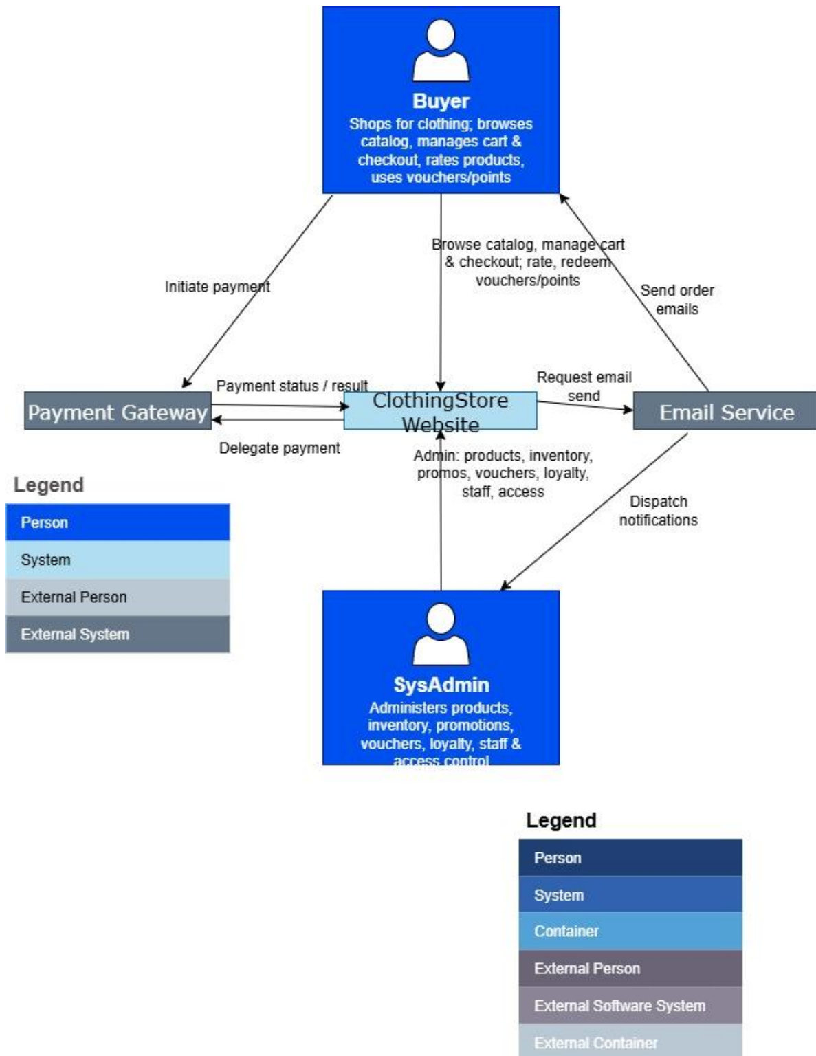
Hình 19. Hình vẽ C1 System Context trong C4 model
