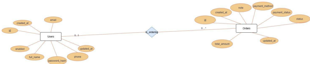
Hình 3. Mối quan hệ ERD giữa bảng User và bảng Order
