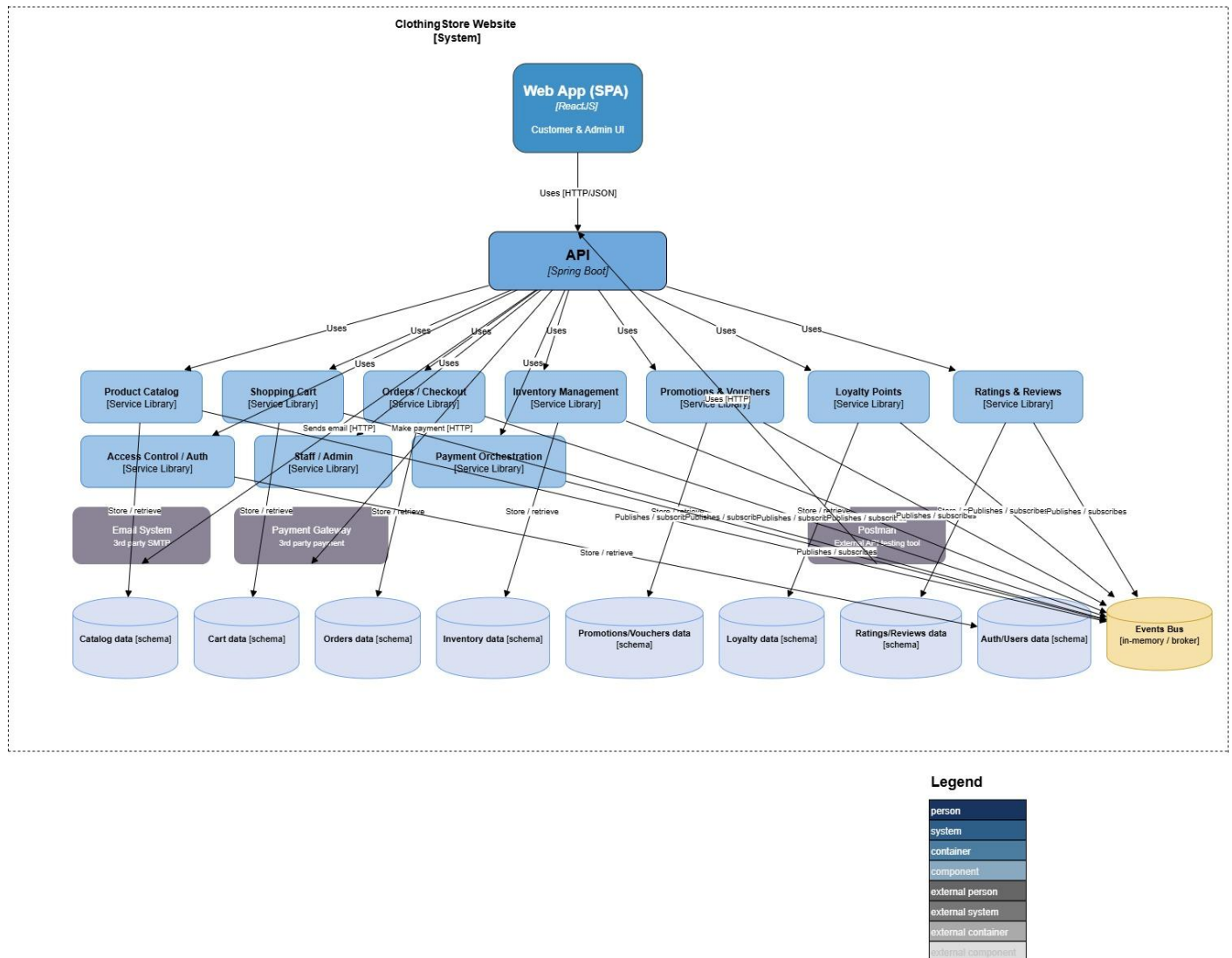
Hình 21. Hình vẽ C3 Component (high-level) trong C4 model
