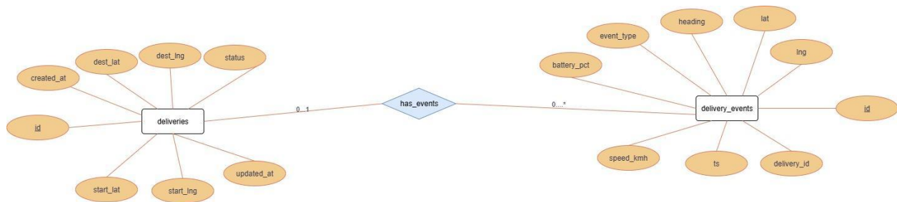
Hình 14. Mối quan hệ ERD giữa bảng Delivery và bảng DeliveryEvent
