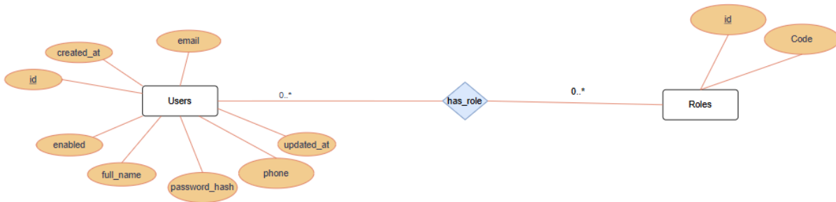
Hình 2. Mối quan hệ ERD giữa bảng User và bảng Role
