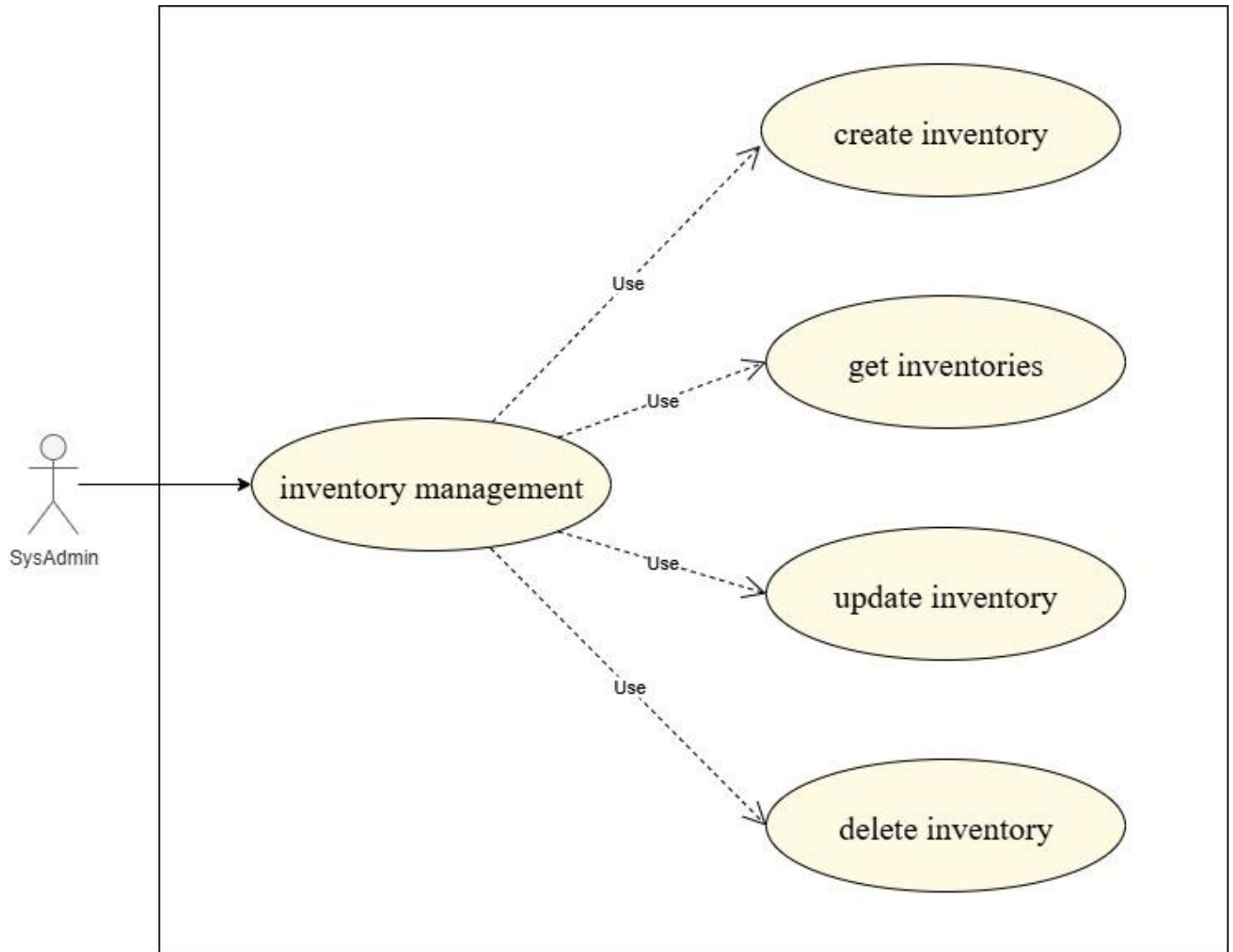
Hình 14. Draw the usecase of Inventory
