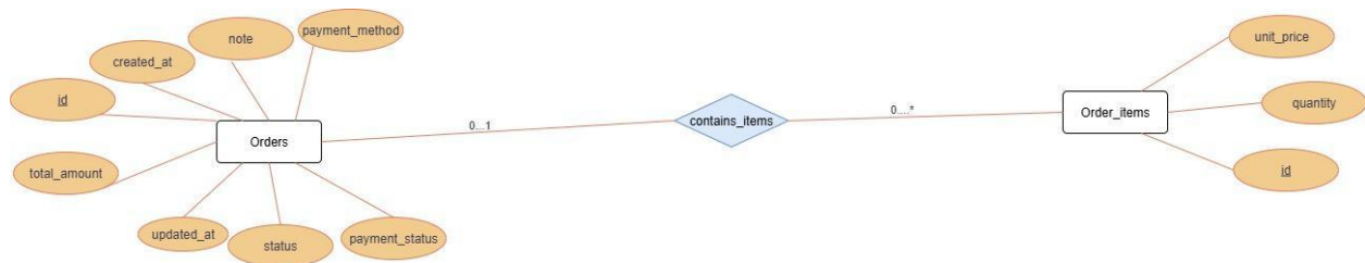
Hình 9. Mối quan hệ ERD giữa bảng Order và bảng OrderItem
