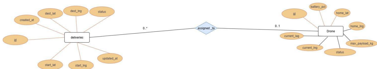
Hình 13. Mối quan hệ ERD giữa bảng Delivery và bảng Drone
