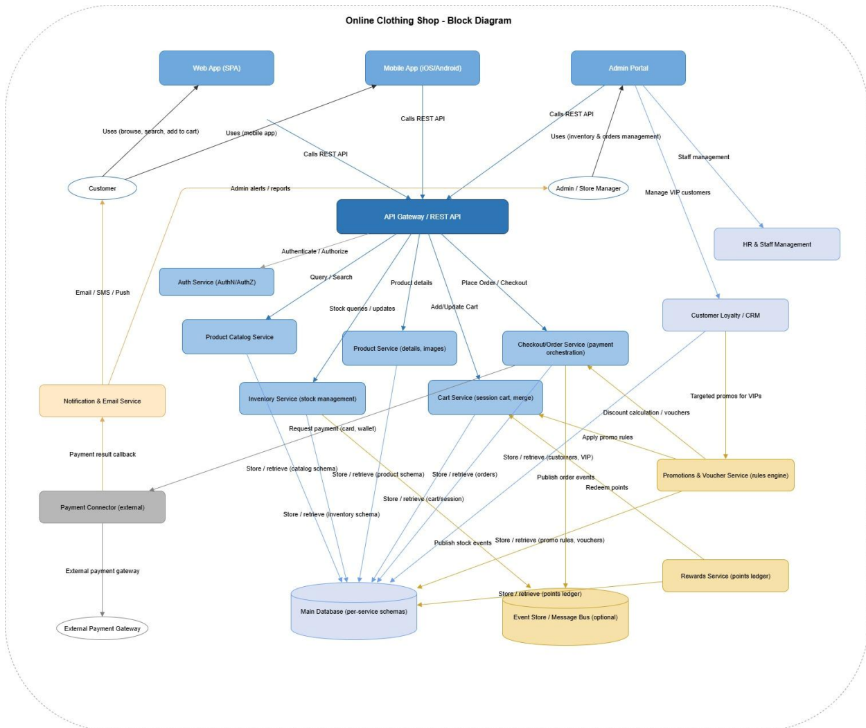
Hình 29. Hình vẽ sơ đồ khối website bán quần áo thời trang
