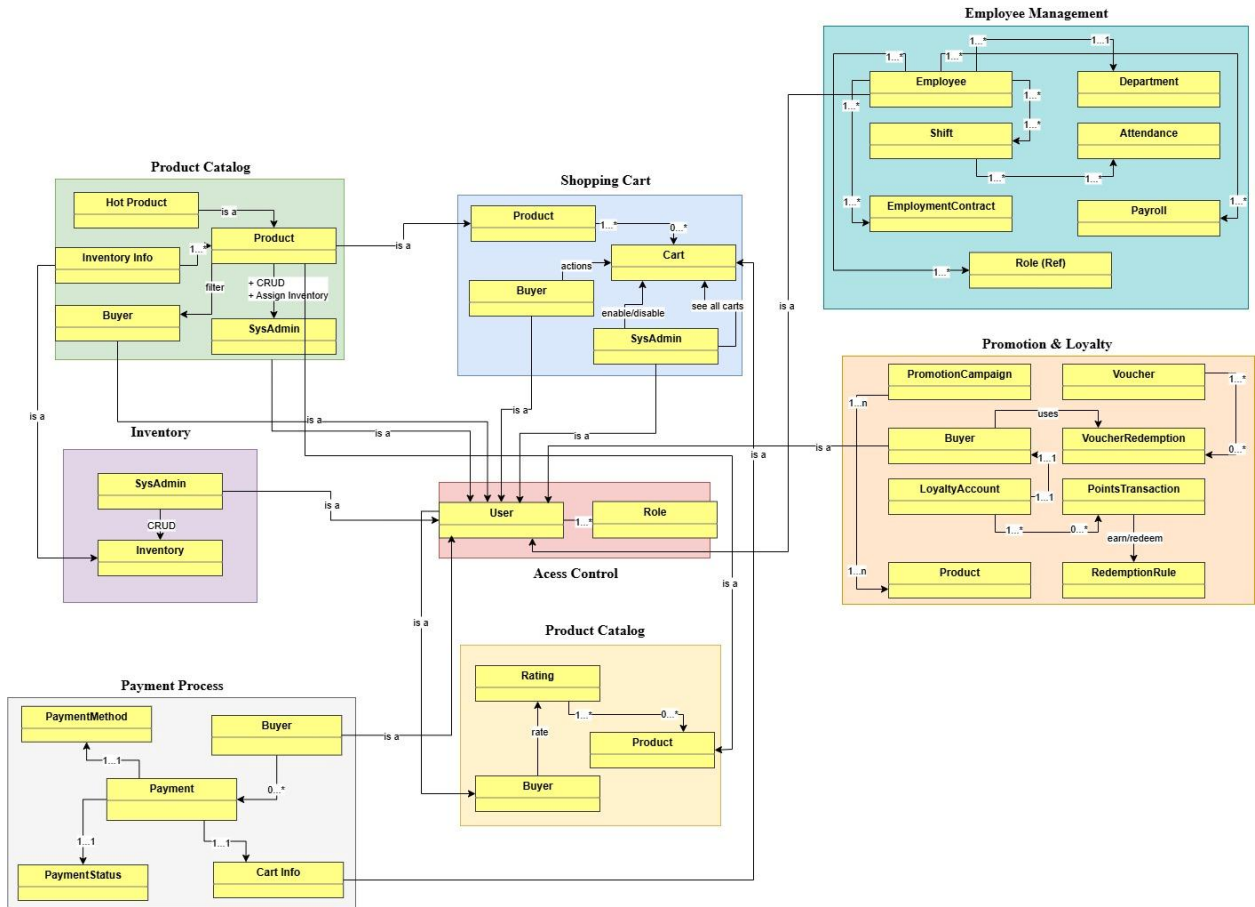
Hình 9. Conceptual Model website bán quần áo thời trang
