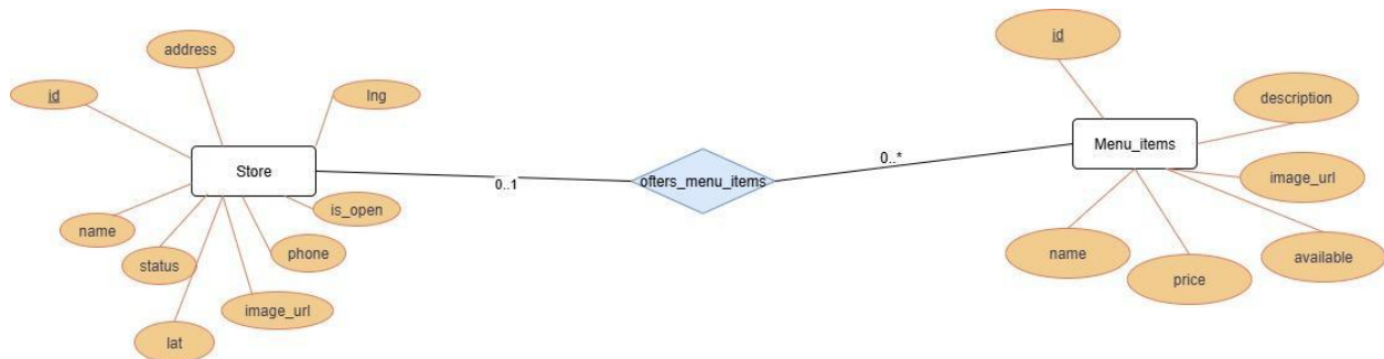
Hình 6. Mối quan hệ ERD giữa bảng Sore và bảng MenuItem
