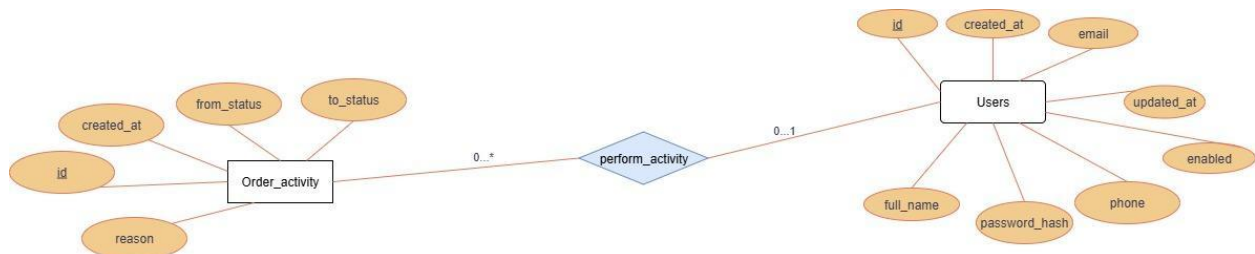
Hình 16. Mối quan hệ ERD giữa bảng OrderActivity và bảng User
