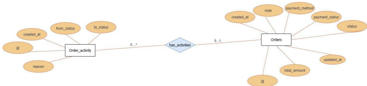
Hình 15. Mối quan hệ ERD giữa bảng OrderActivity và bảng Order
