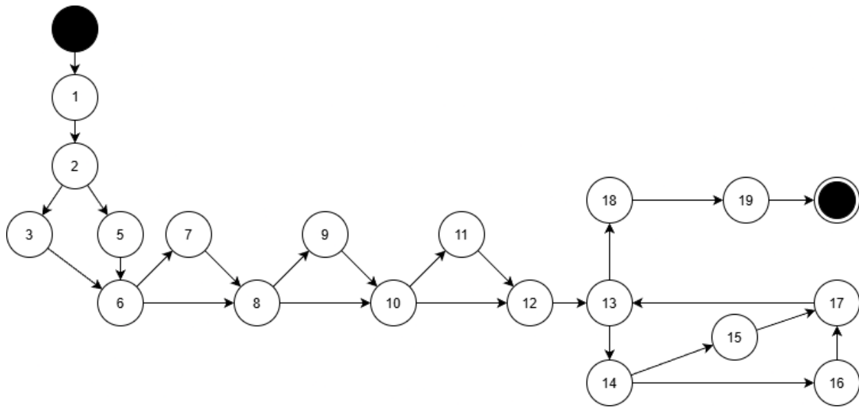
Hình 39. Đồ thị dòng điều khiển của Kiểm thử hộp trắng
