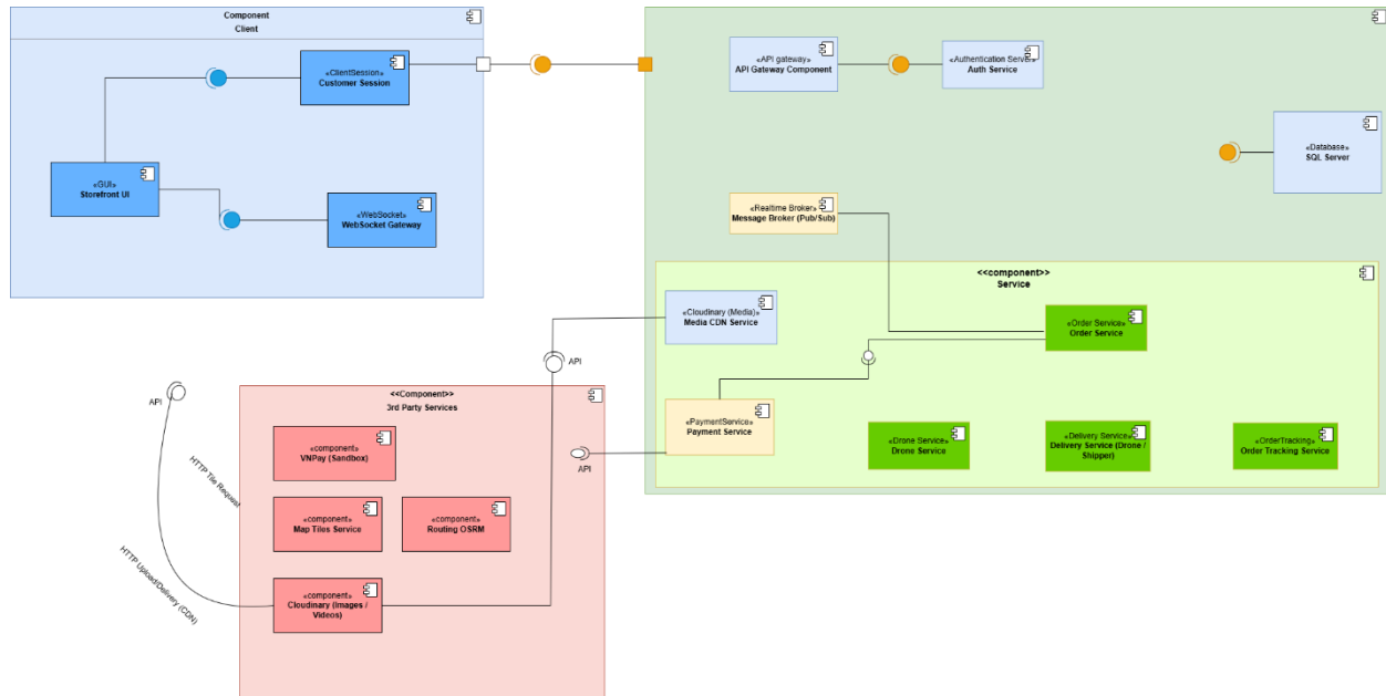
Hình 28. Component Clients/Customers Server
