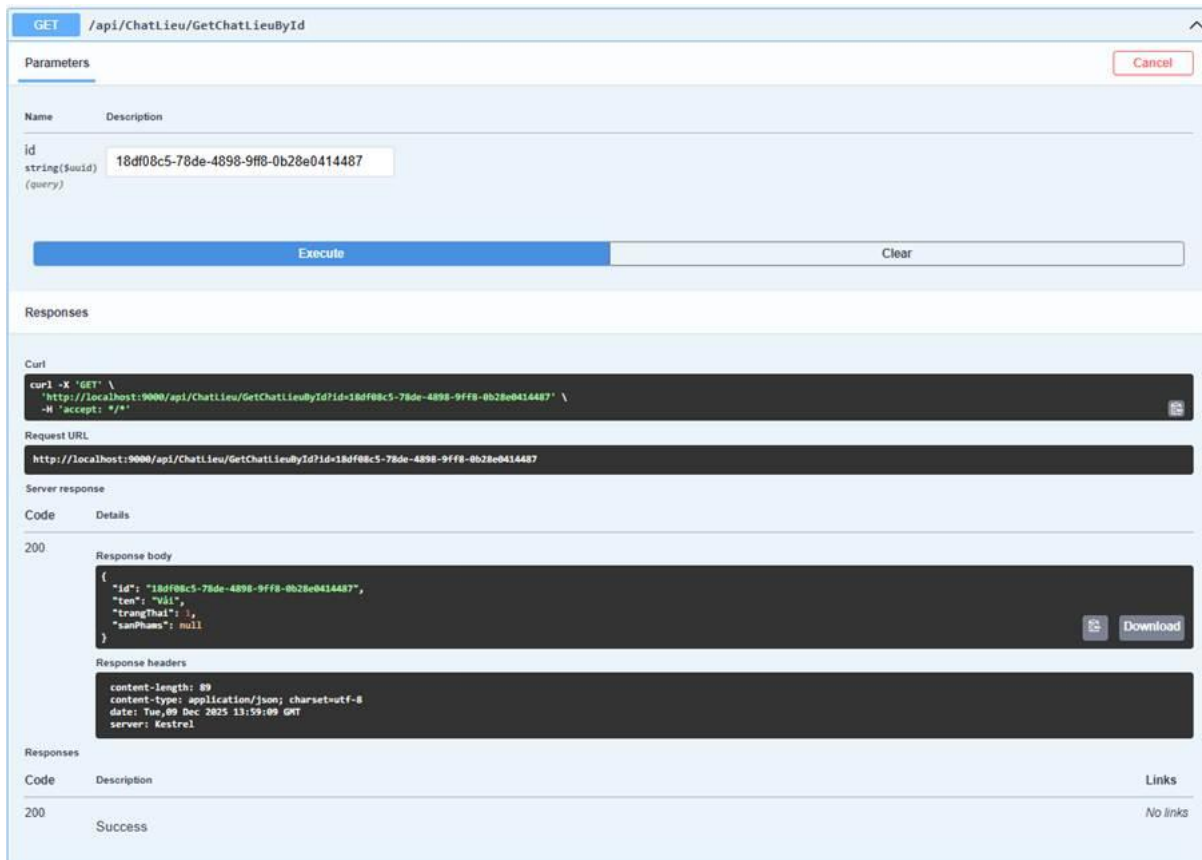
Hình 36. Kiểm thử thủ công cho API bằng Swagger
