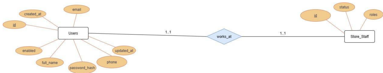
Hình 4. Mối quan hệ ERD giữa bảng User và bảng StoreStaff
