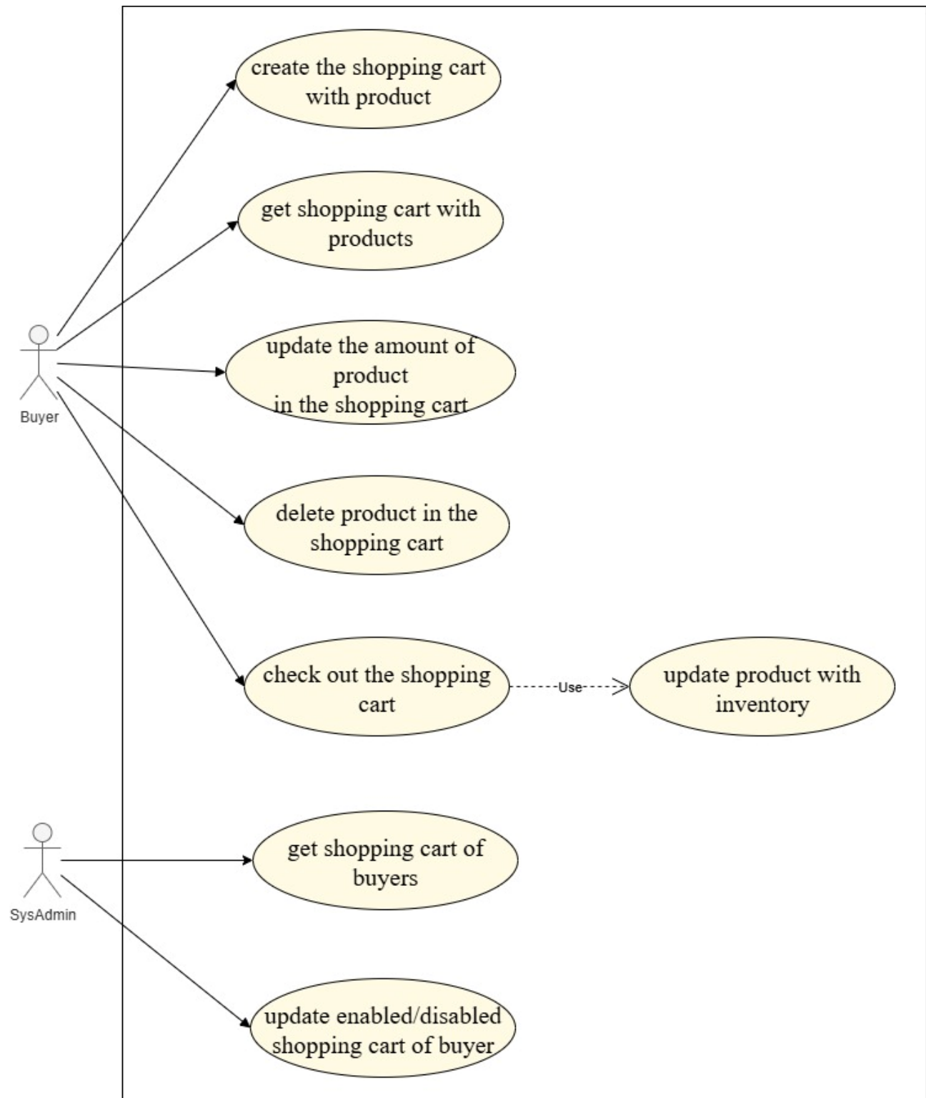
Hình 12. Draw the usecase of Shopping Cart
