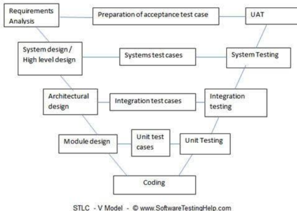
Hình 35. Hình ảnh tổng quan về V-model
