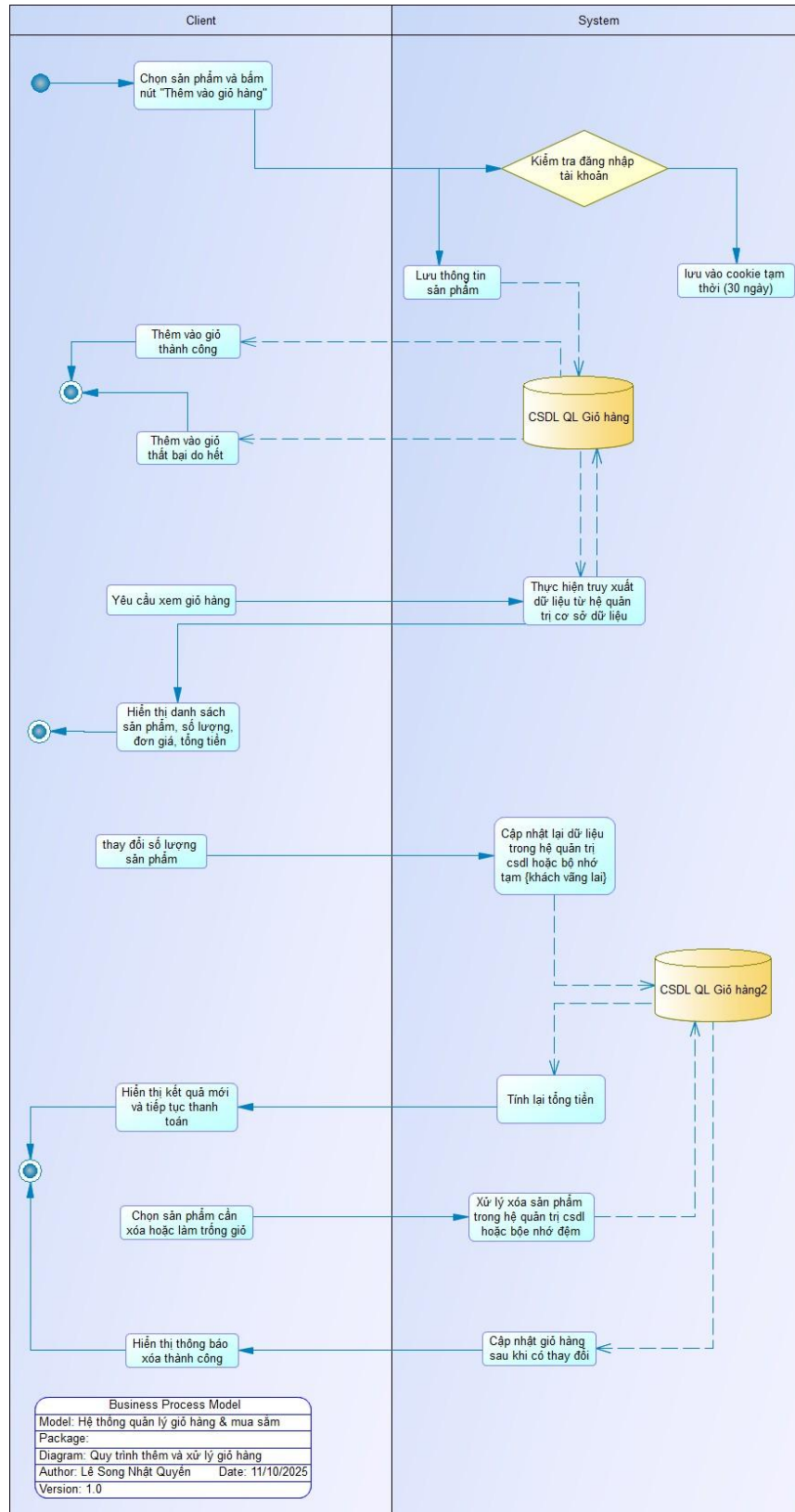
Hình 2. Quy trình thêm và xử lý giỏ hàng
